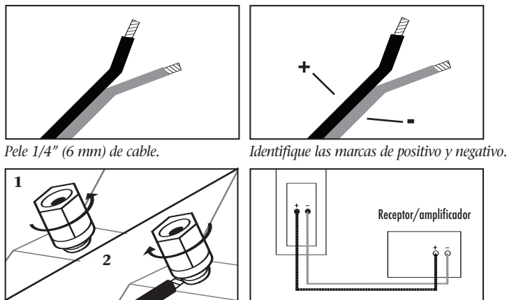
Figura 2: conexión de cables y polaridad
