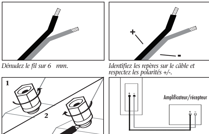
Figure 2 – Câblage et polarité
