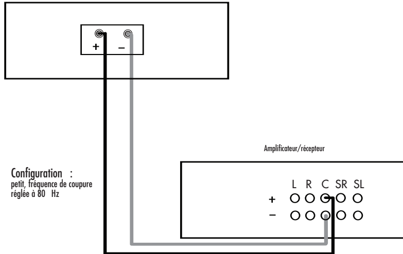
Figure 3 – Raccorder l'enceinte à l'amplificateur
