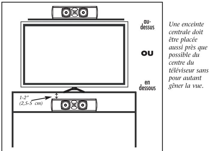
Figure 1 – Positionnement de l'enceinte centrale Série CS
