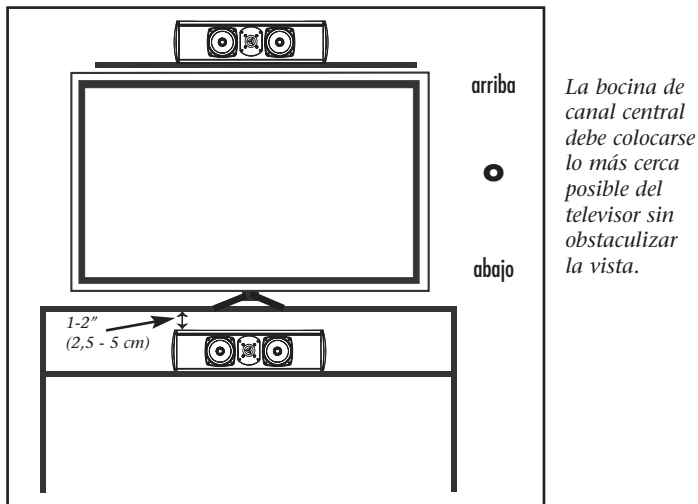
Figura 1: colocación del canal central de la serie CS
