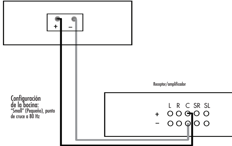
Figura 3: conexión de la bocina al amplificador
