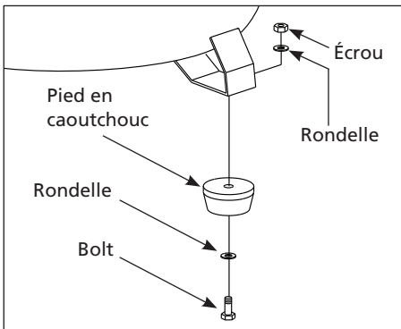
Figure 1 - Pied en caoutchouc de montage
