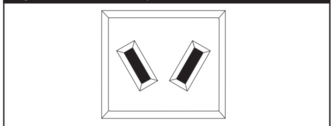
Figure 29 - Prise de 10 Ampères, 12 Volts c.c.
