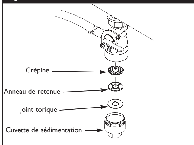
Figure 32 — Entretien de la Vanne de Combustible
