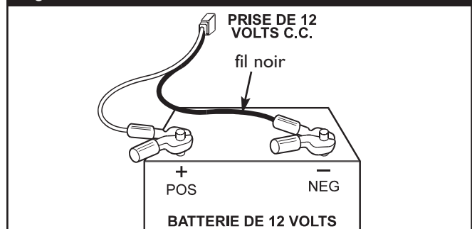
Figure 23 - Branchement des Câbles de Batterie
