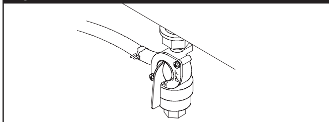
Figure 20 - Robinet d'arrivée d'essence
