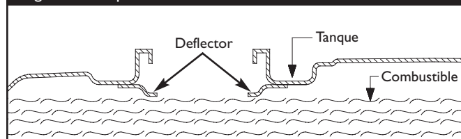
Figura 34 - Espacio de Combustible
