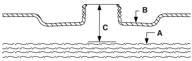
Figura 2 – Expansión del Combustible A - Combustible B - Tanque de Combustible C - Espacio de Tanque
