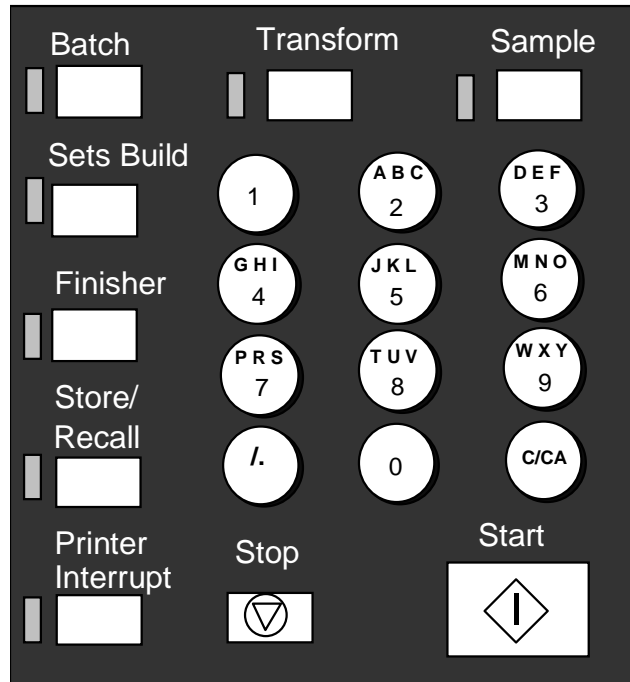
Numeric Keypad
