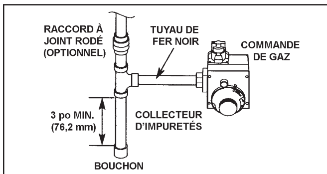
FIGURE 21 – TUYAUTERIE DE GAZ EN FER NOIR MENANT À LA COMMANDE DE GAZ
