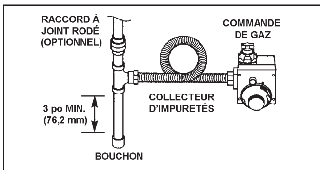
FIGURE 20 – TUYAUTERIE DE GAZ AVEC RACCORD FLEXIBLE
